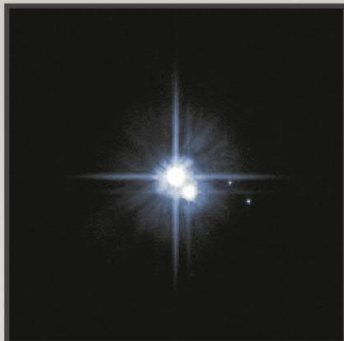
A Plútó földi távcsővel Pluto through an Earth-based telescope
