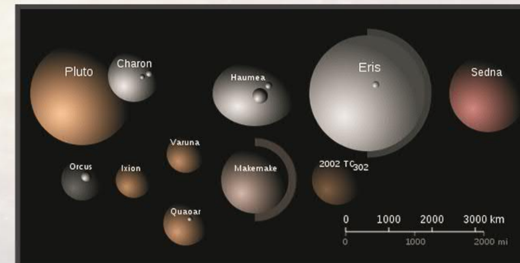
A Kuiper-öv nagyobb égitestjei, a plutonidák Major celestial bodies of the Kuiper belt: the plutoids
